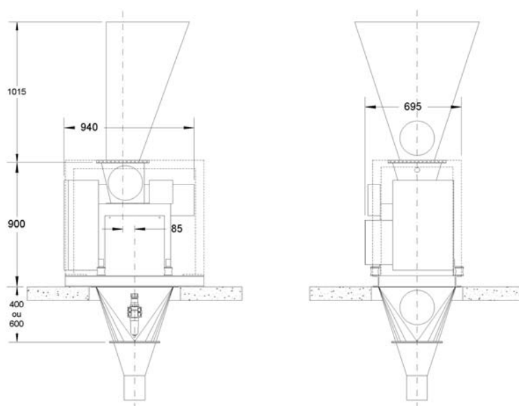
Doseuse pondérale "JANOMATIC Gr/15-é" pour ensachage de produits granuleux.
